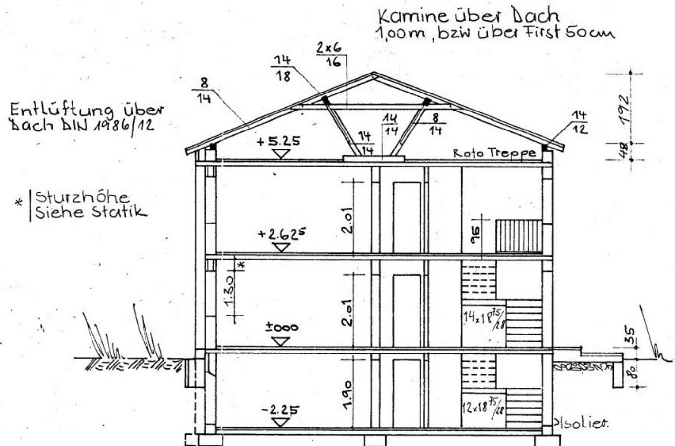
SCHNITT WOHNHAUS
