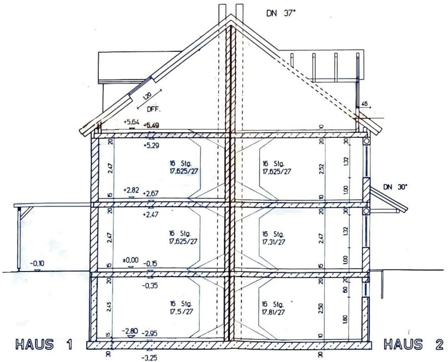
Schnitt A-A
